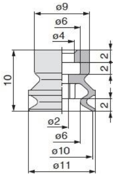
ZP3-10B□ (重量 : 0.8 g)
