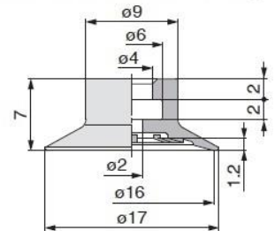
ZP3-16UM (重量：0.8 g)
