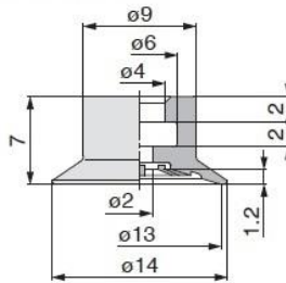
ZP3-13UM (重量：0.7 g)
