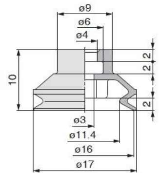
ZP3-16B□ (重量 : 1.1 g)
