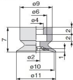
ZP3-10UM (重量：0.6 g)
