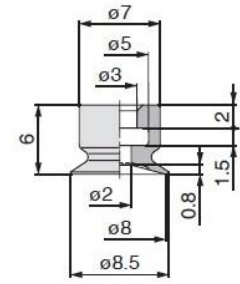
ZP3-08UM (重量：0.3 g)
