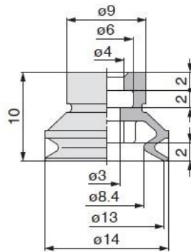
ZP3-13B□ (重量 : 1.0 g)
