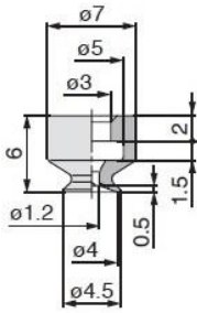
ZP3-04UM (重量：0.3 g)
