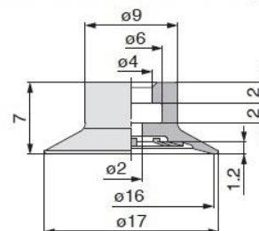
ZP3-16UM (重量：0.8 g)
