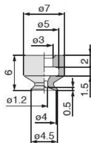
ZP3-04UM (重量：0.3 g)
