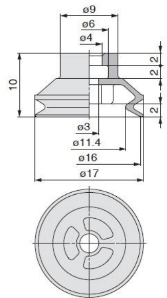
ZP3-16B□ (重量 : 1.1 g)
