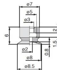
ZP3-08UM (重量：0.3 g)
