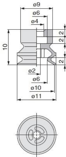
ZP3-10B□ (重量 : 0.8 g)
