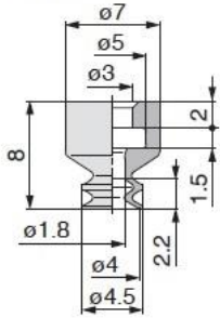
ZP3-04B□ (重量 : 0.3 g)
