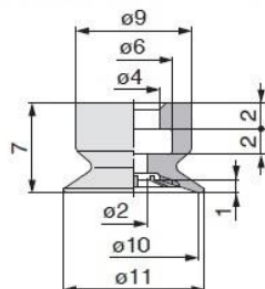
ZP3-10UM (重量：0.6 g)
